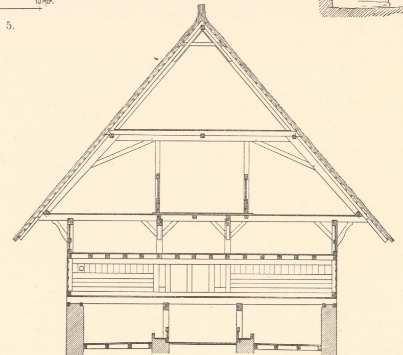
Abb. 5. Einbach. Schnitt C D (des Grundrisses auf Blatt Baden No. 6).
