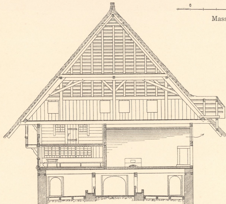
Abb. 4. Einbach. Schnitt B C (des Grundrisses auf Blatt Baden No. 6)
