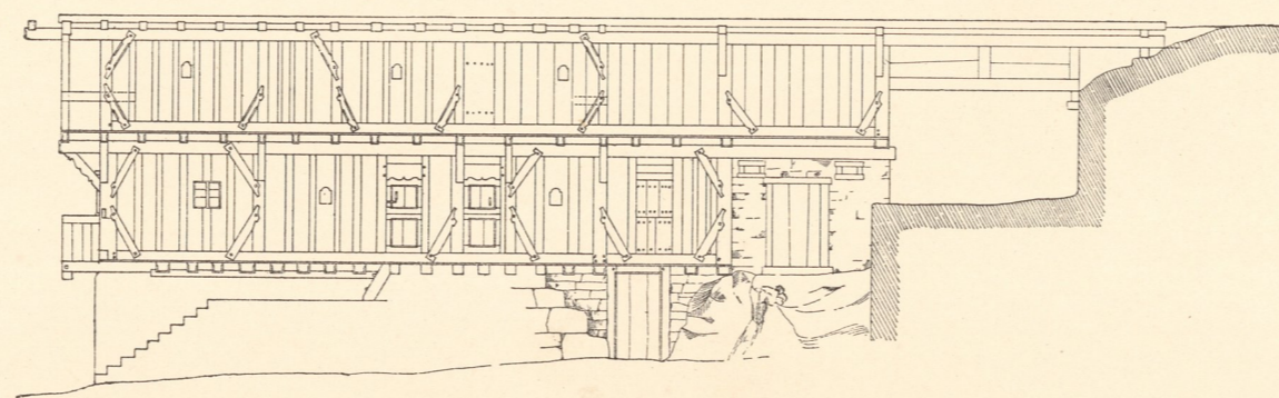
Abb. 7. Simmersbachthal. Längenschnitt C D.
