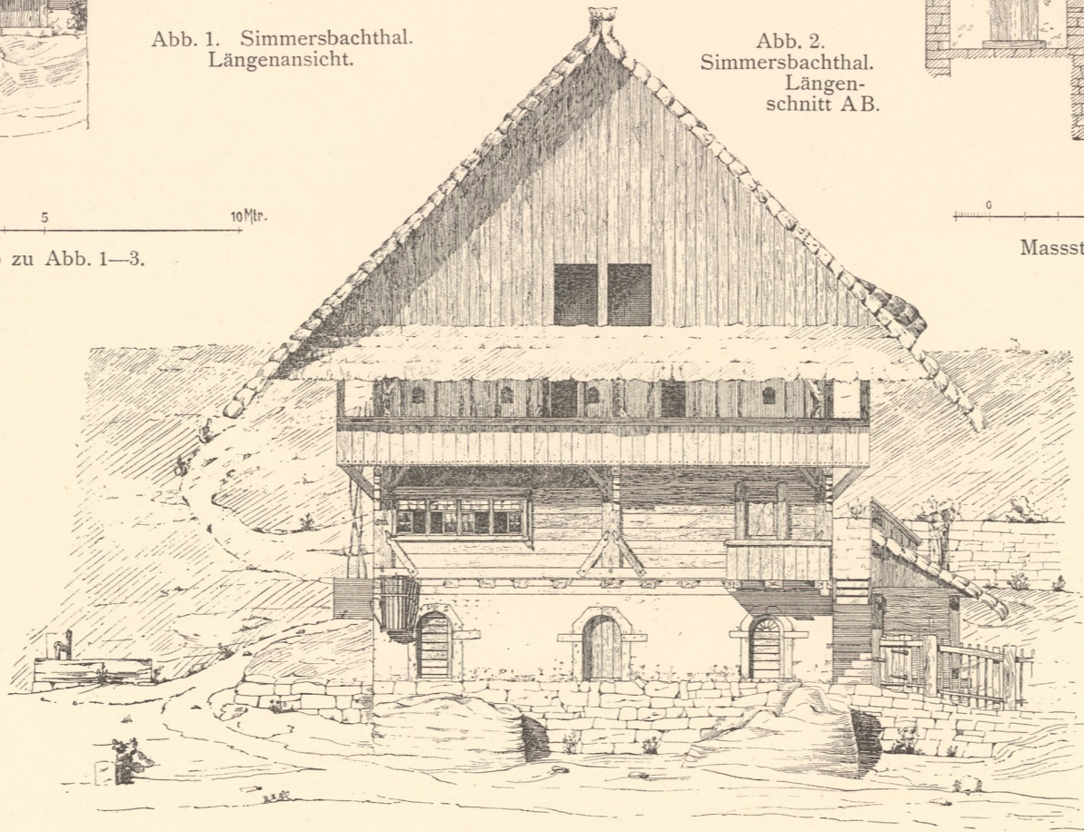
Abb. 3. Simmersbachthal. Giebelansicht.
