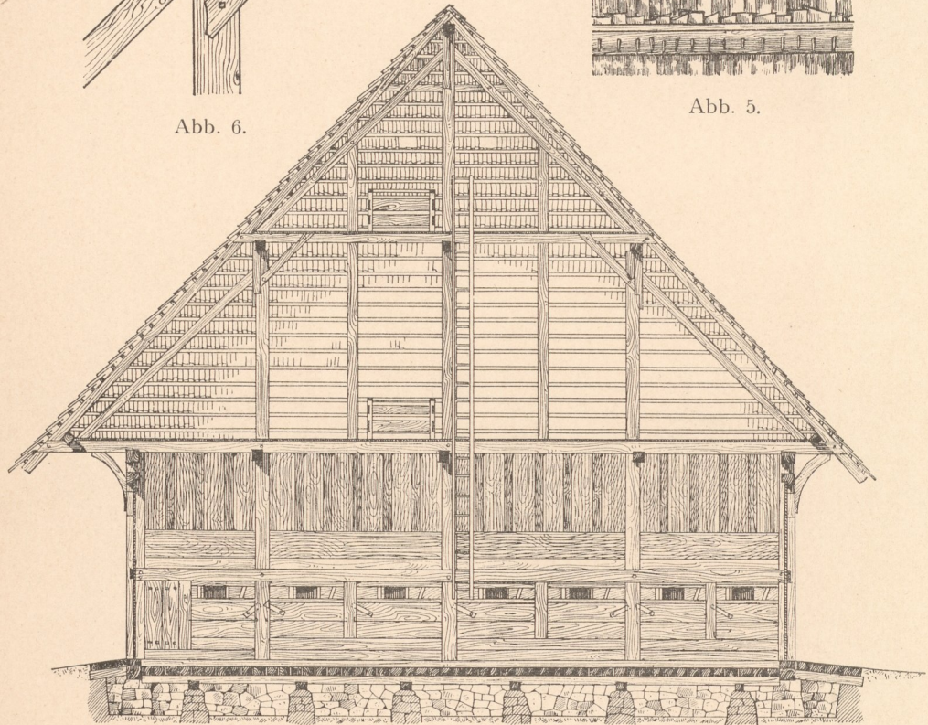
Abb. 3. Querschnitt B C.
