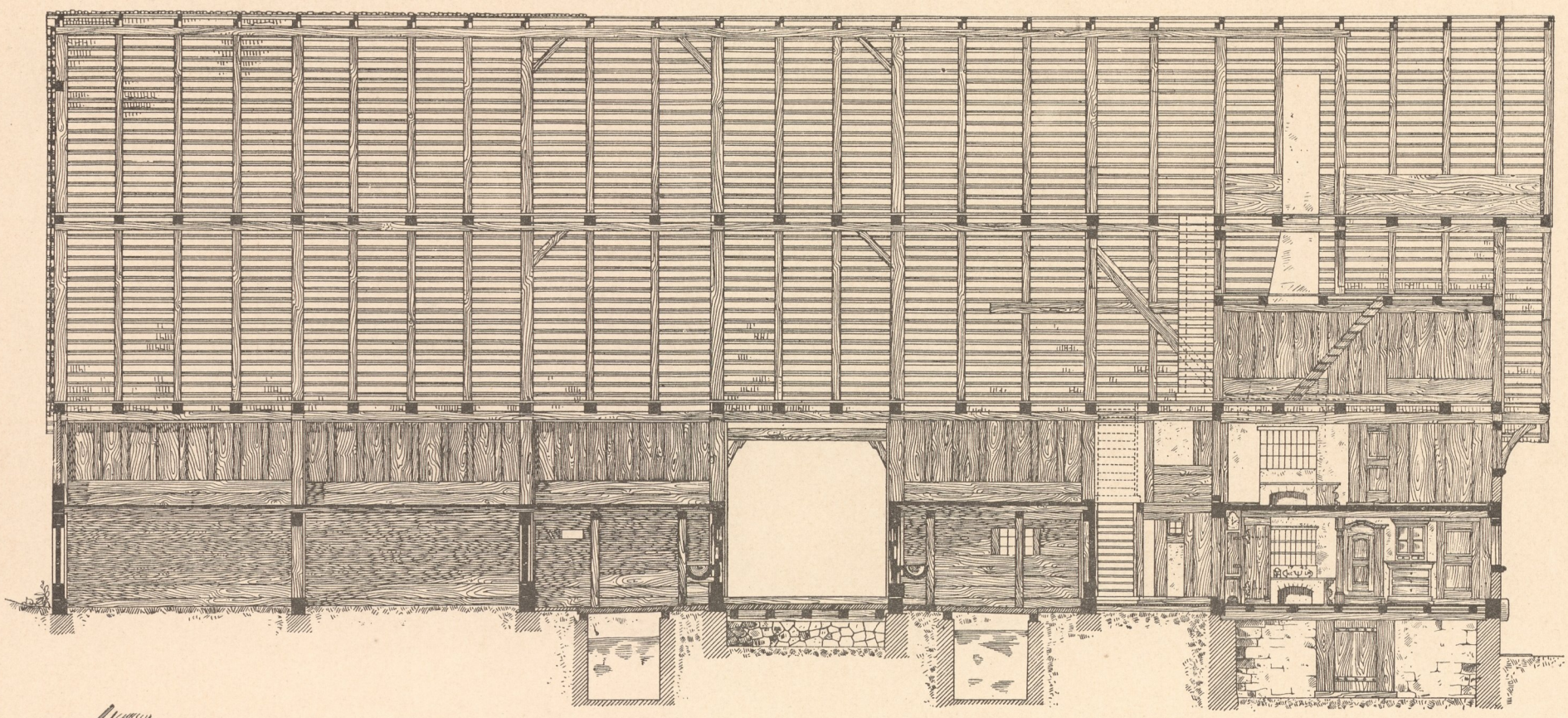
Abb. 2. Längenschnitt.
