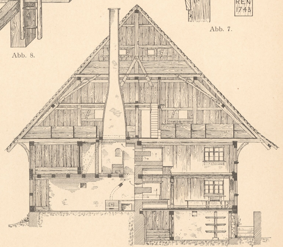
Abb. 4. Querschnitt A B.
