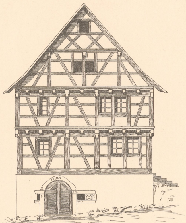
Abb. 1. Giebelansicht.
