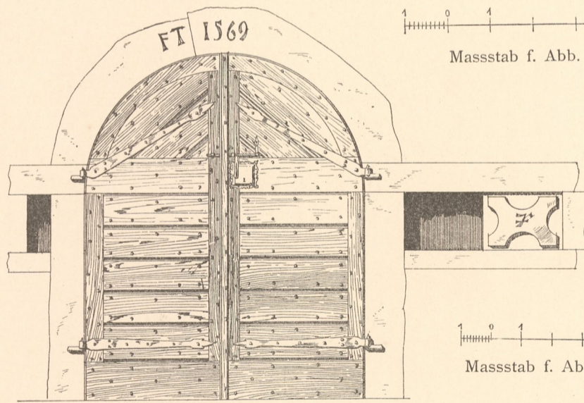
Abb. 8. Kellerthür.
