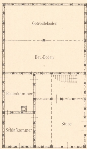
Abb. 5. Grundriss vom Obergeschoss.
