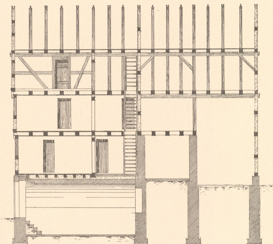
Abb. 3. Längenschnitt.
