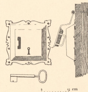
Abb. 10. Schloss an der Kellerthür.
