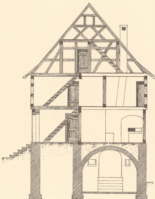
Abb. 4. Querschnitt.
