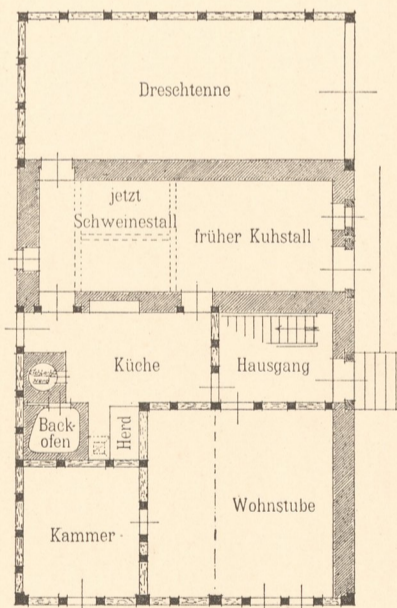
Abb. 6. Grundriss vom Erdgeschoss.
