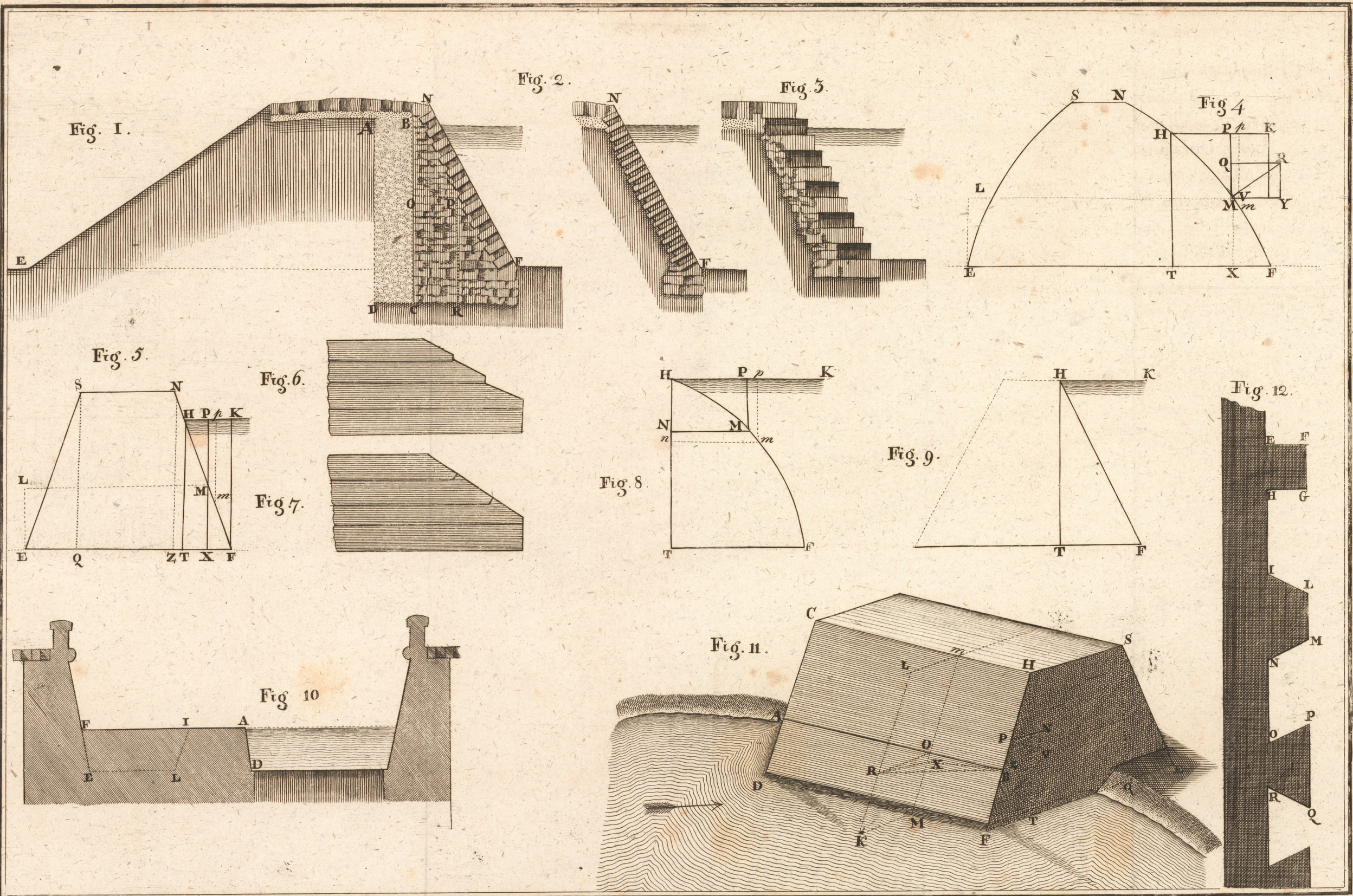
1 2 3 4 5 6 Fuß Maßstab zu Fig. 1. 2 und 3 2 Toisen
