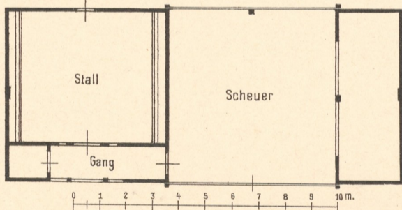
Grundriss zum Wirtschaftsgebäude in Trnava.
