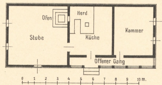
Grundriss zum Wohnhaus Nr. 25.
