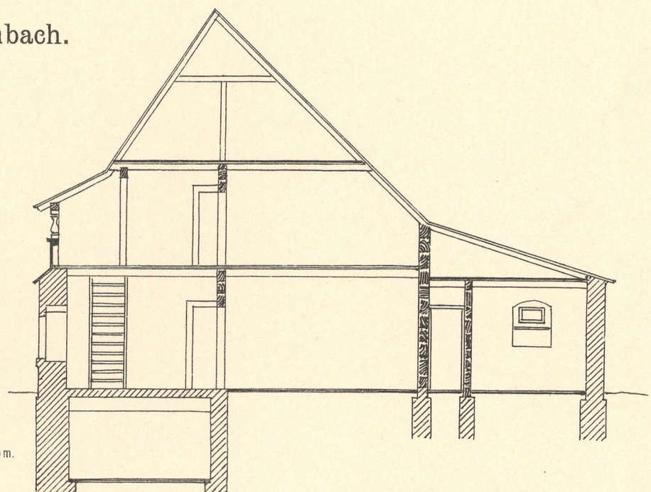
Querschnitt.
