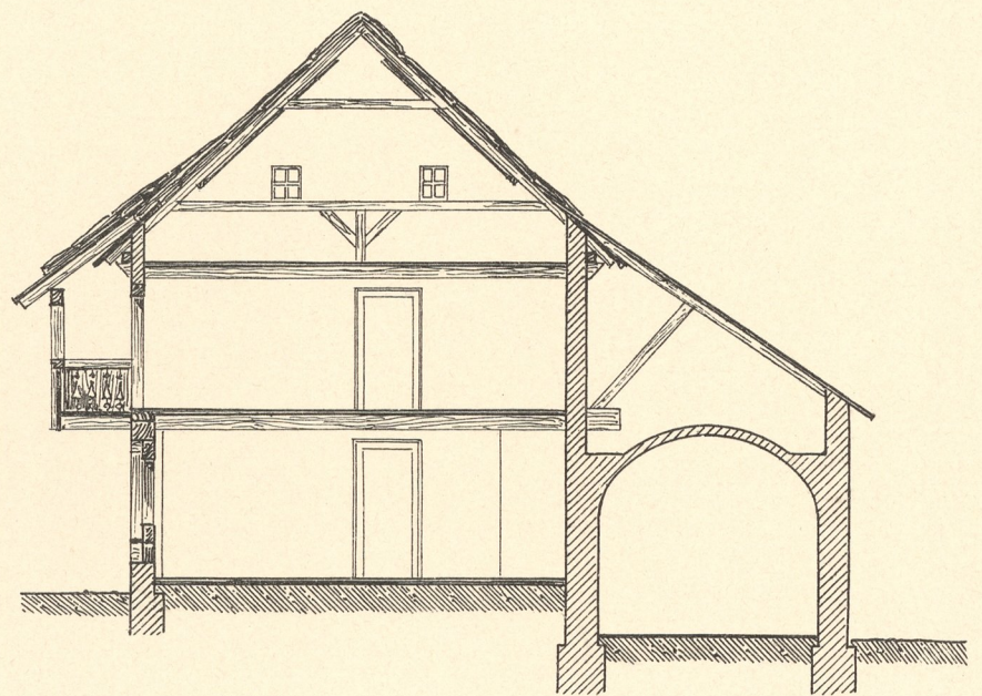
Querschnitt.
