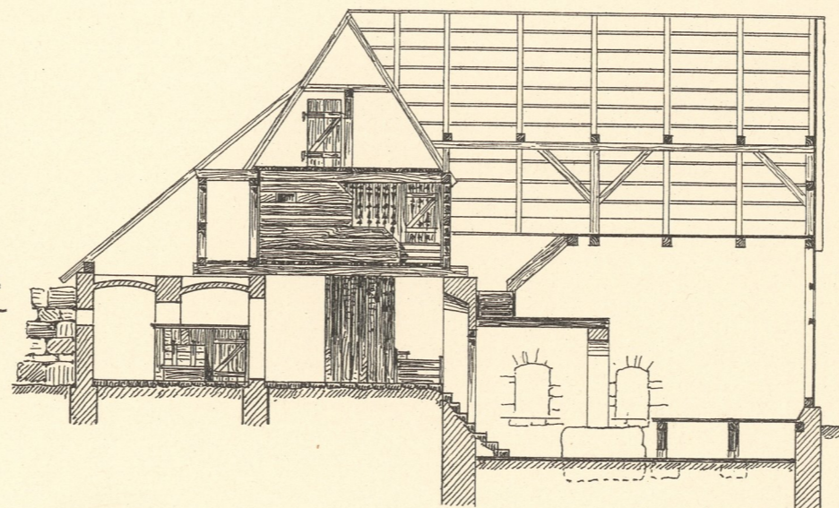
Längsschnitt.
