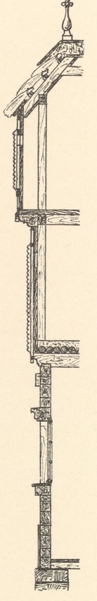
Schnitt.
