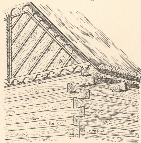
Detailzeichnung.
