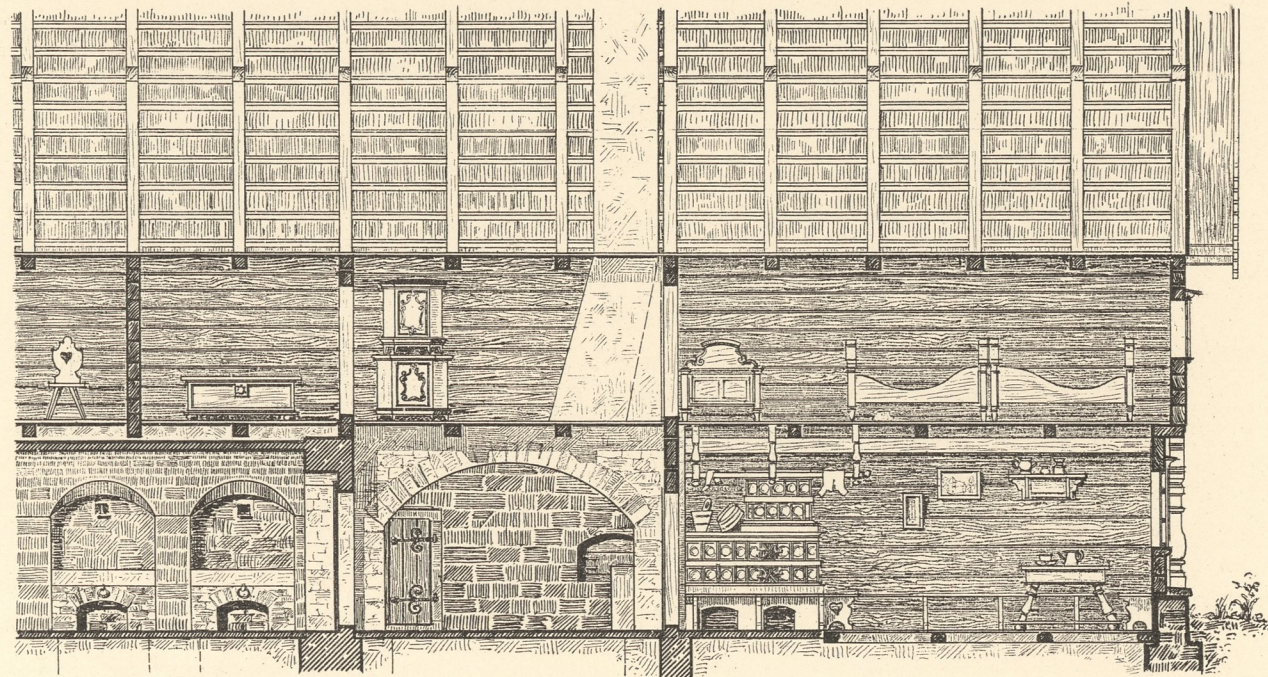
Längenschnitt A B.
