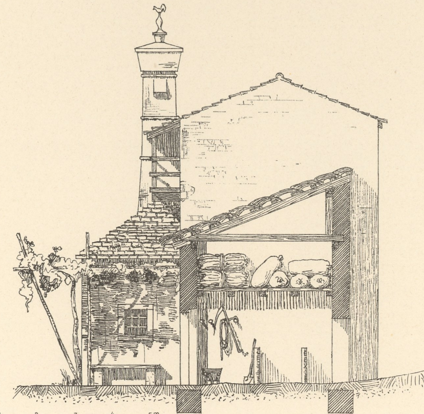
Seitenansicht.
