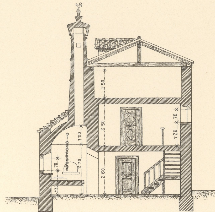
Querschnitt.
