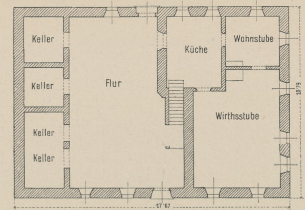
Grundriss.
