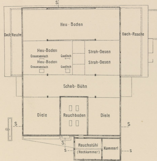
Ebenerd-Geschoss.
