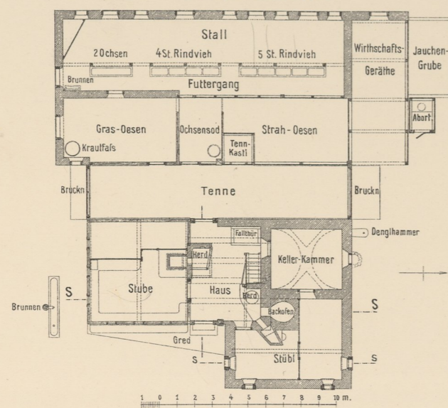
Ebenerd-Geschoss.
