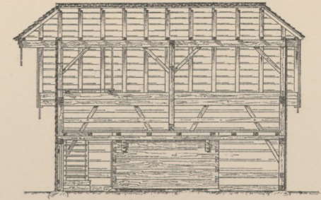
Längsschnitt ss.
