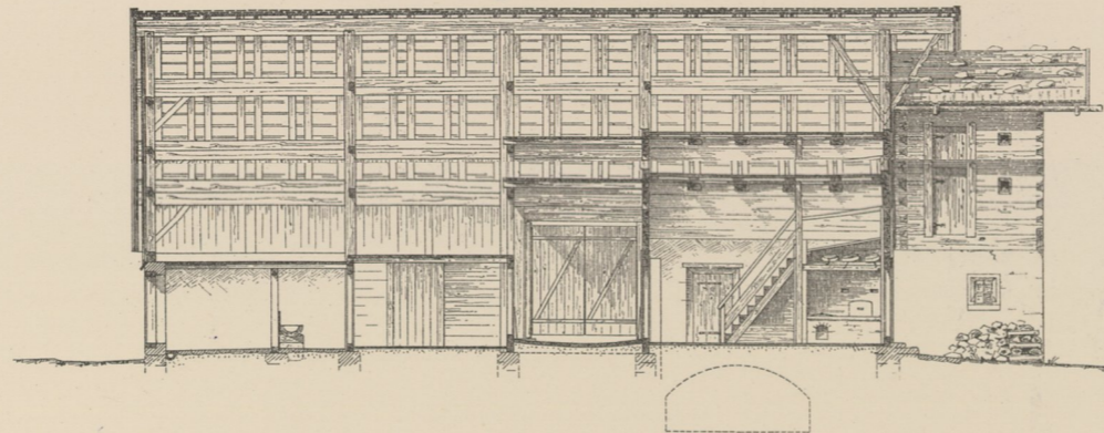
Querschnitt ss.
