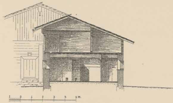
Schnitt ss durch den Vorbau.
