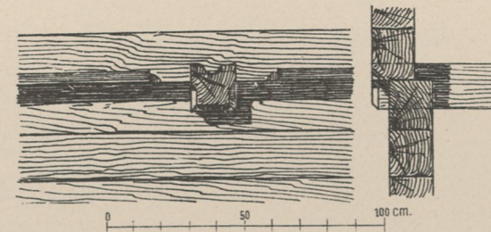
Detail vom Hofwirth-Haus in Raab, 1786.
