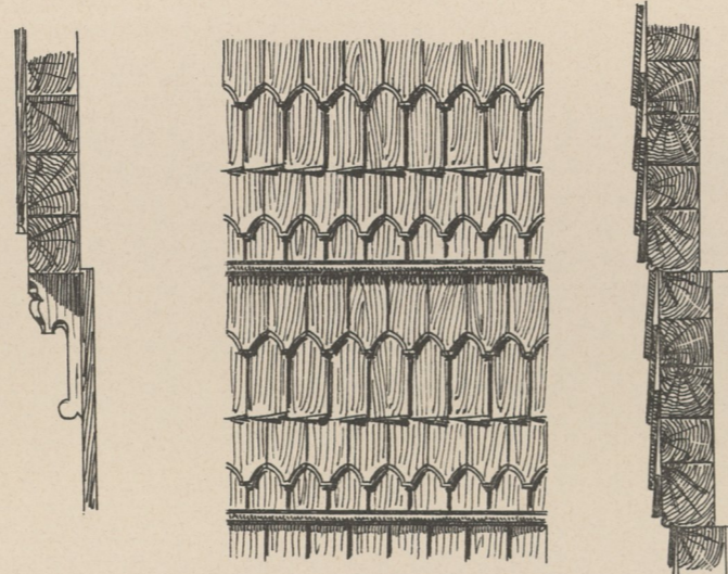
Beschindelung der Blockwände am Doctorhaus in Siegharting.
