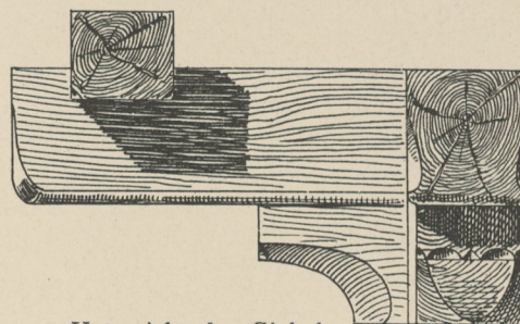
Untersicht der Giebel-Console.
