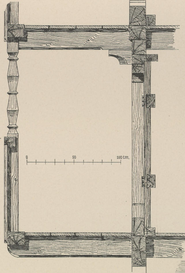
Detail des Balkons vom Getreidekasten des Schwarzmeiergutes in Siegharting.
