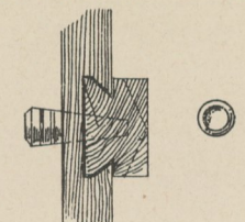
Detail der Holznägel an der Getreidekastenthür.
