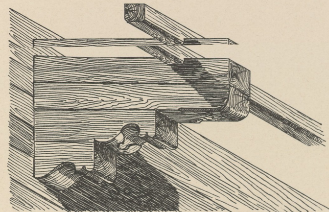
Console vom Doctorhaus in Siegharting 1780.
