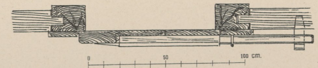
Stock der Balkonthüre von der Mühle zu Steegen bei Peuerbach.
