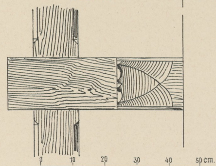
Untersicht der Giebel-Console.
