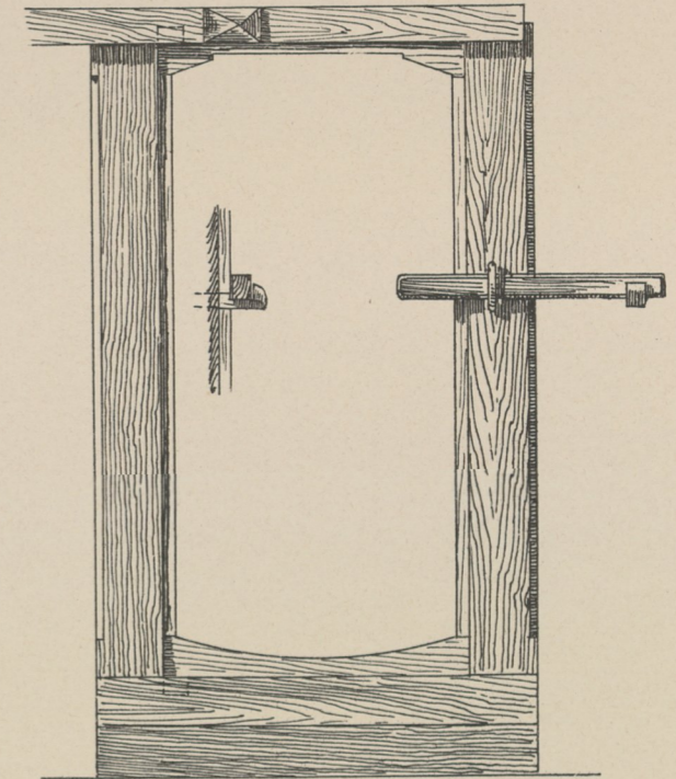
Stock der Balkonthüre von der Mühle zu Steegen bei Peuerbach.
