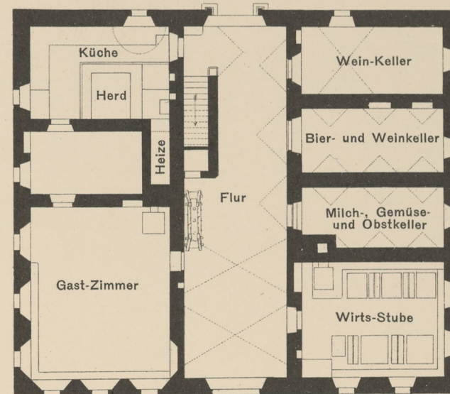
Parterre-Grundriss.
