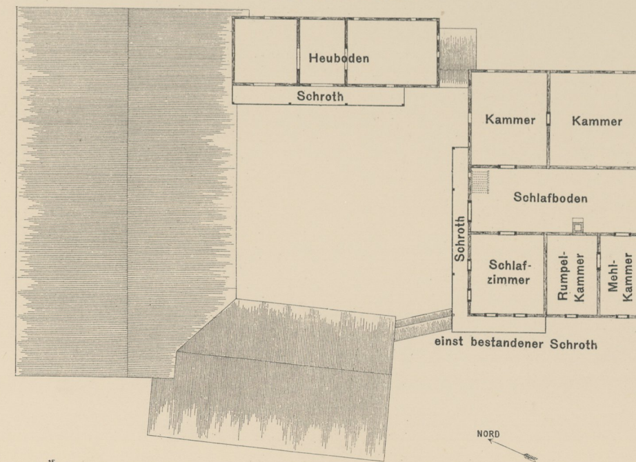
I. Stock-Grundriss.
