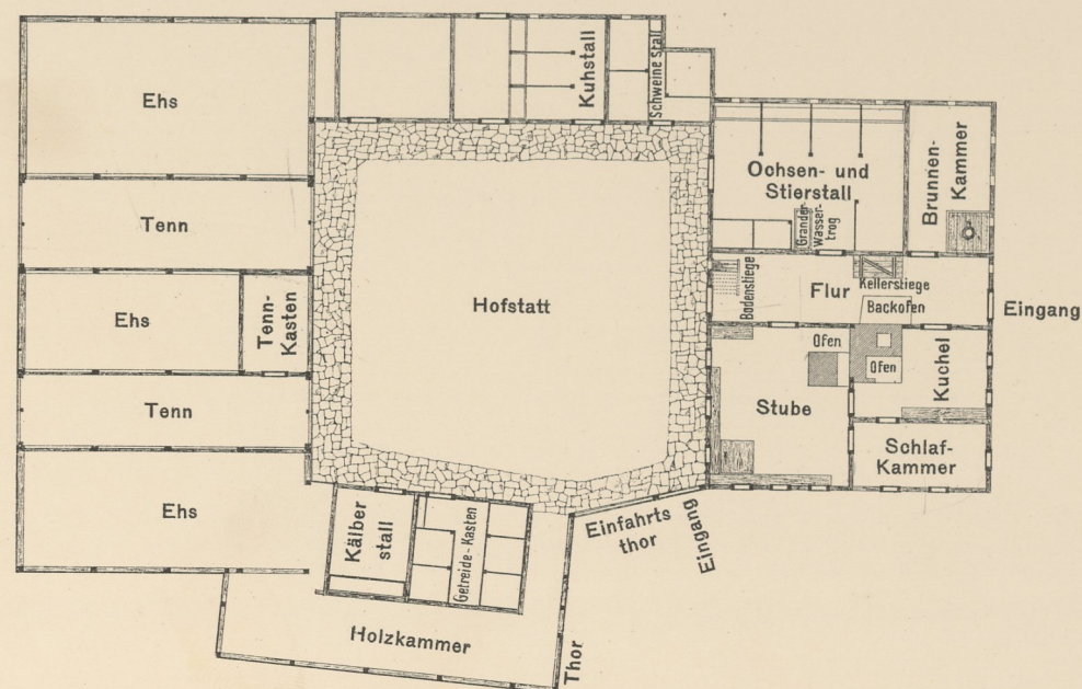
Parterre-Grundriss.
