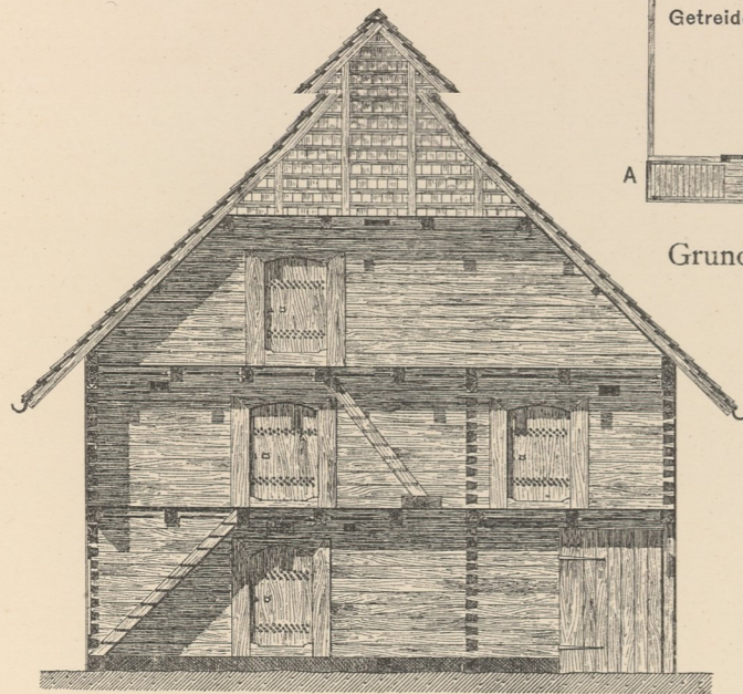
Schnitt A B.
