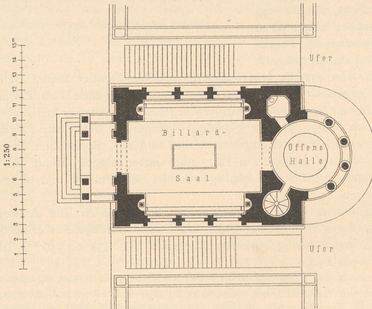
Fig. 436. Grundriss.
