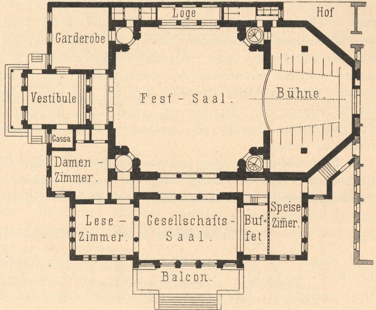
Fig. 345. Hauptgeschoss.
