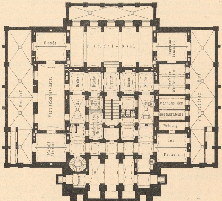
Fig. 346. Sockelgeschoss.
