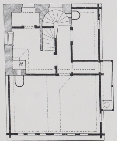
Grundriss der I Etage.
