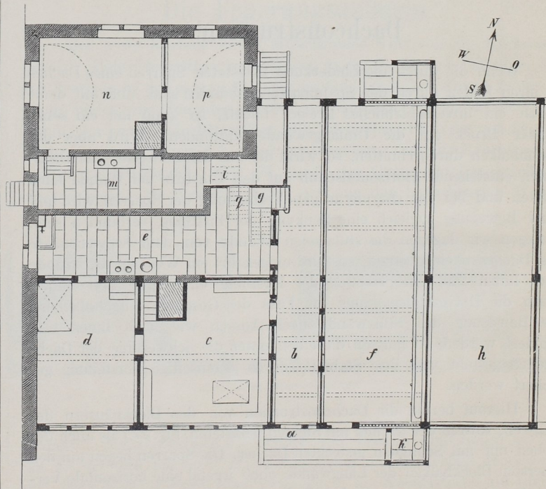
Fig. 24. Maasstab 1 : 200.
