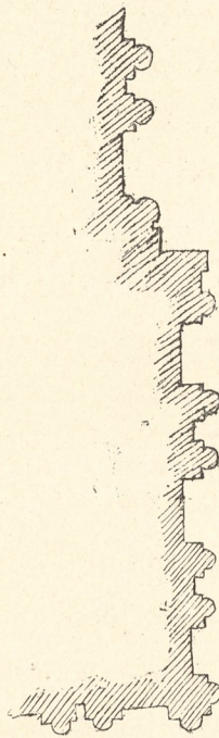
Fig. 89. — Angle extérieur des talars et retombée des grands arcs.
