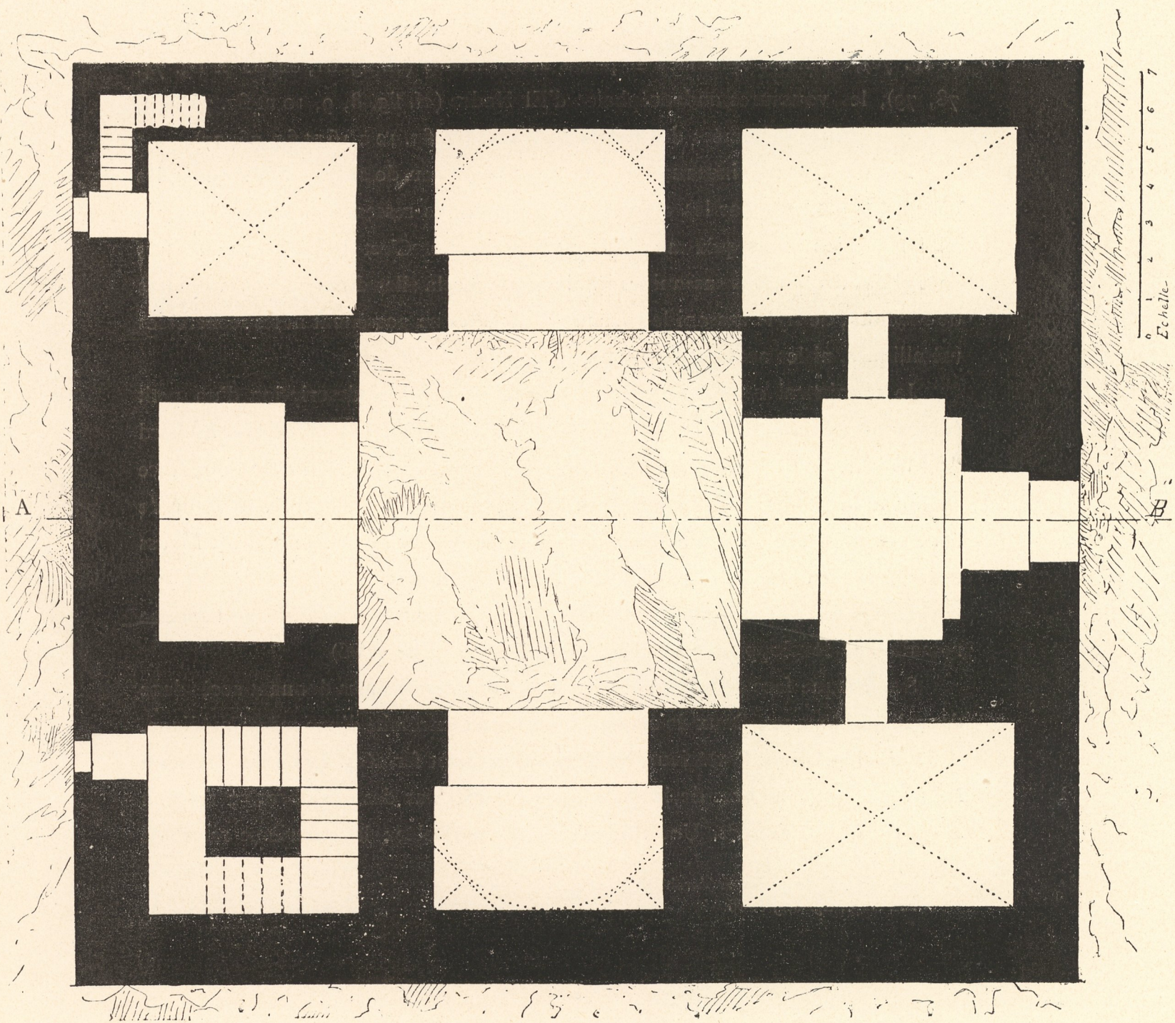
Fig. 85. — Monument de Rabbath-Ammân : Plan.
