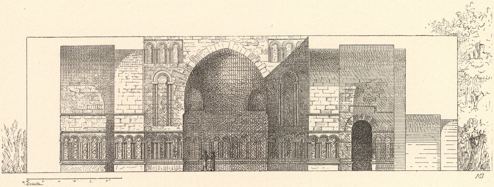
Fig. 84. — Coupe transversale A B.
