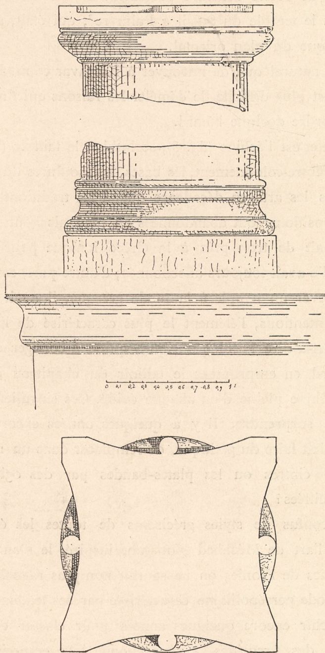
Fig. 3, 4 et 5. — Détails du chapiteau, de la base des colonnes et de la corniche du stylobate du temple de Kingavar.
