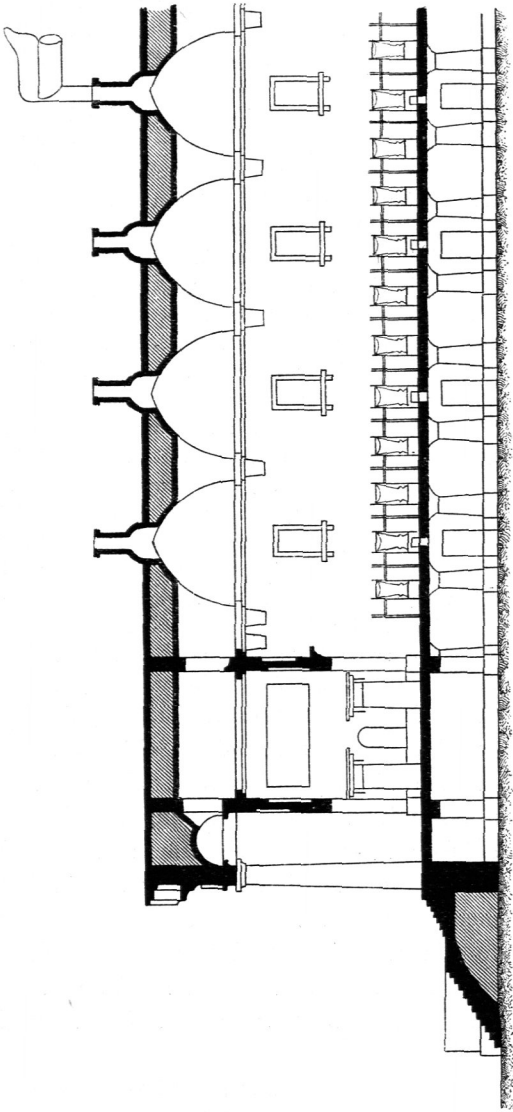
Fig. 25. Längenschnitt.
