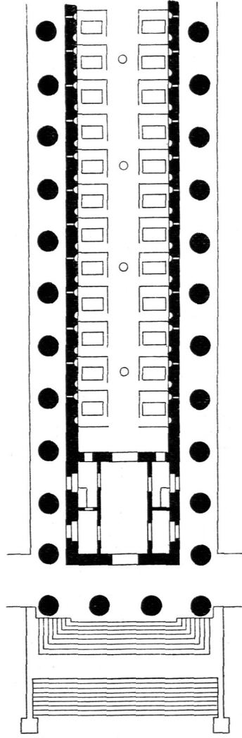
Fig. 26. Grundriß.
