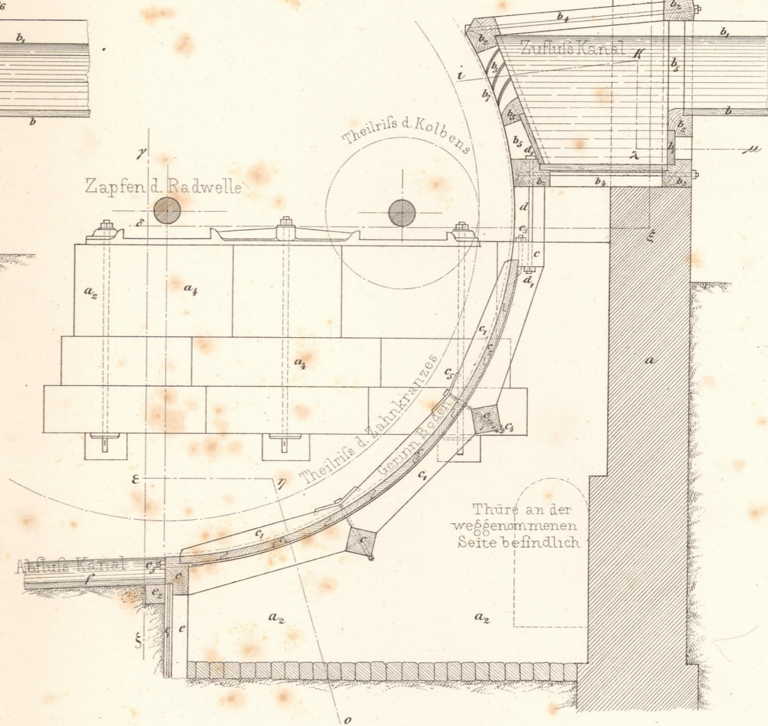
Fig. 4. Horizontal-Durchschnitt des Einlaufes nach i κ λ μ
