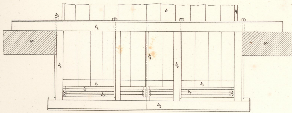
Fig. 3. Horizontal Ansicht des Einlaufes.
