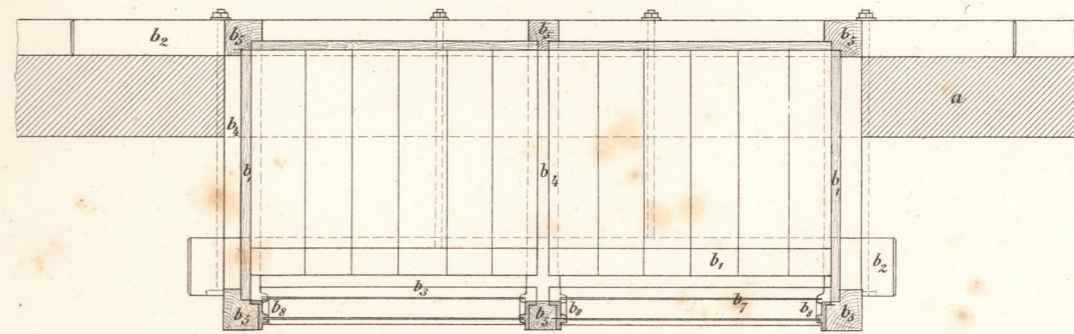
Fig. 4. Horizontal-Durchschnitt des Einlaufes nach i κ λ μ
