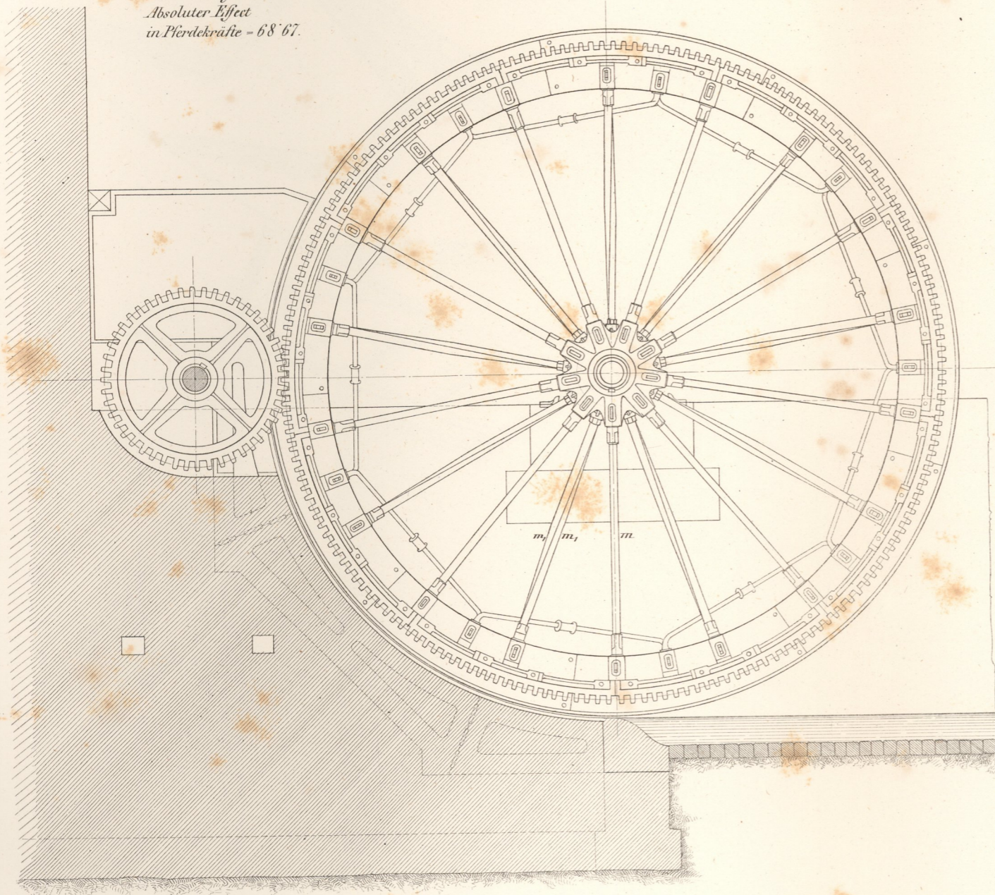
Fig 1 Ansicht des Rades.
