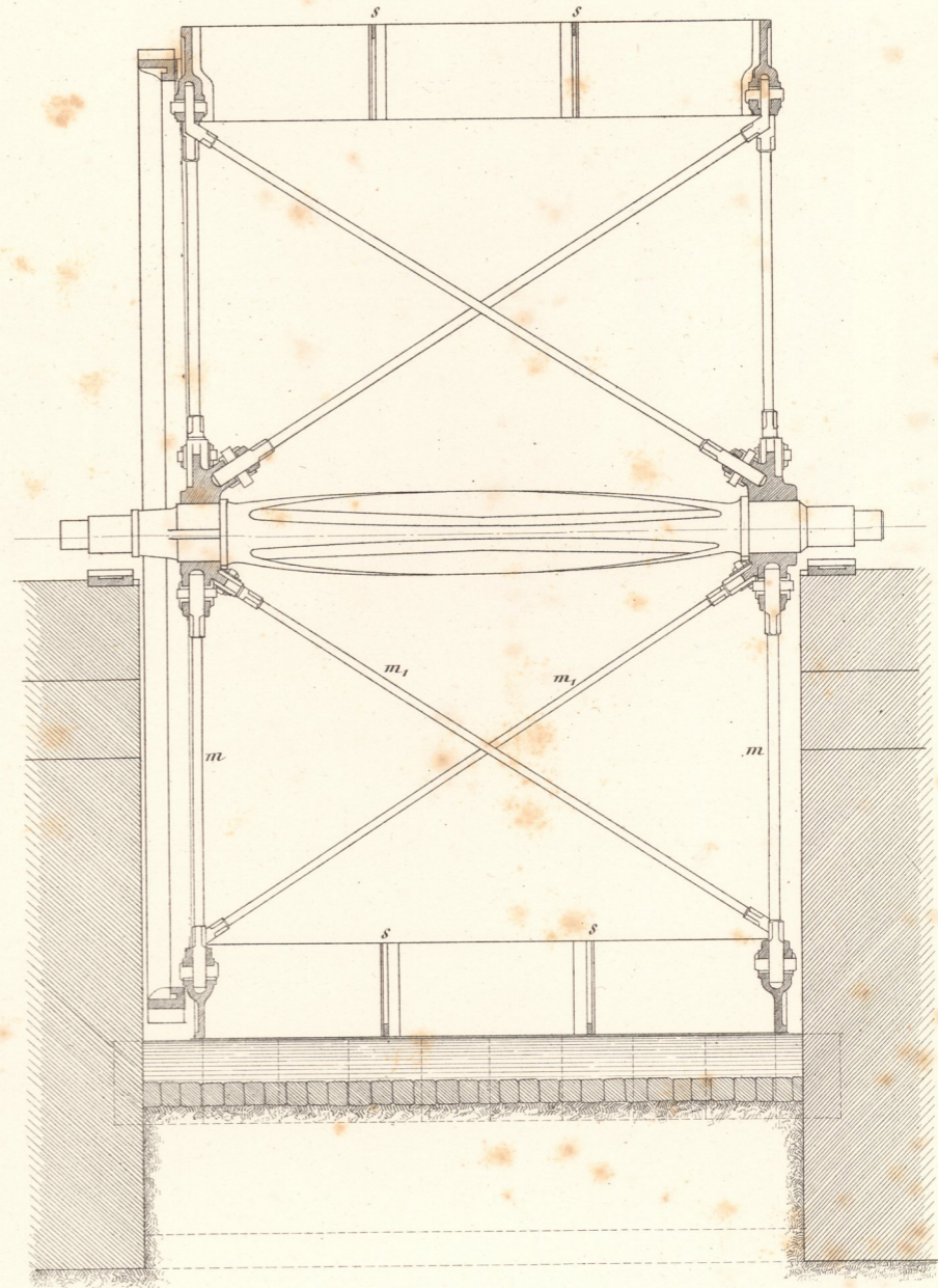
Fig. 2 Vertikal Durchschnitt des Rades.
