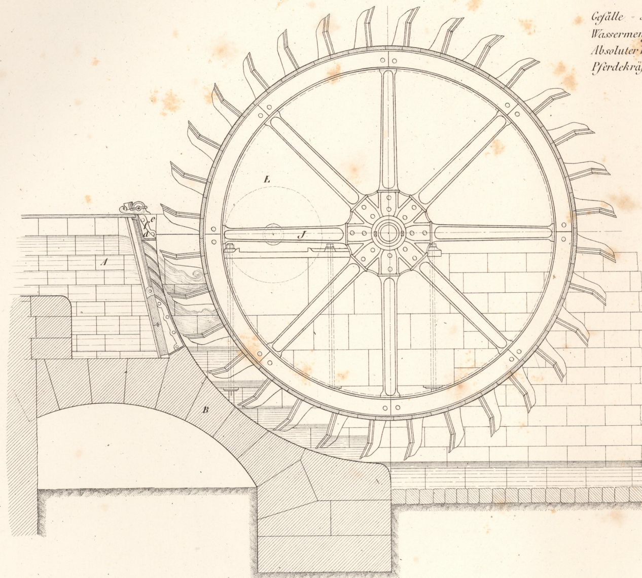
Fig. 1. Ansicht des Rades und Durchschnitt des Gerinnes.
