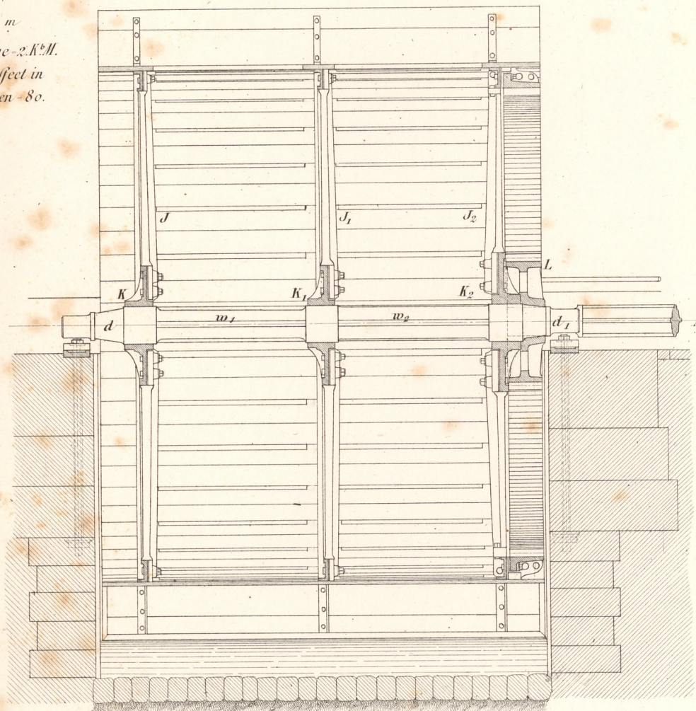
Fig. 2. Vertikal-Schnitt durch das Rad und durch die Gerinn-Mauer.
