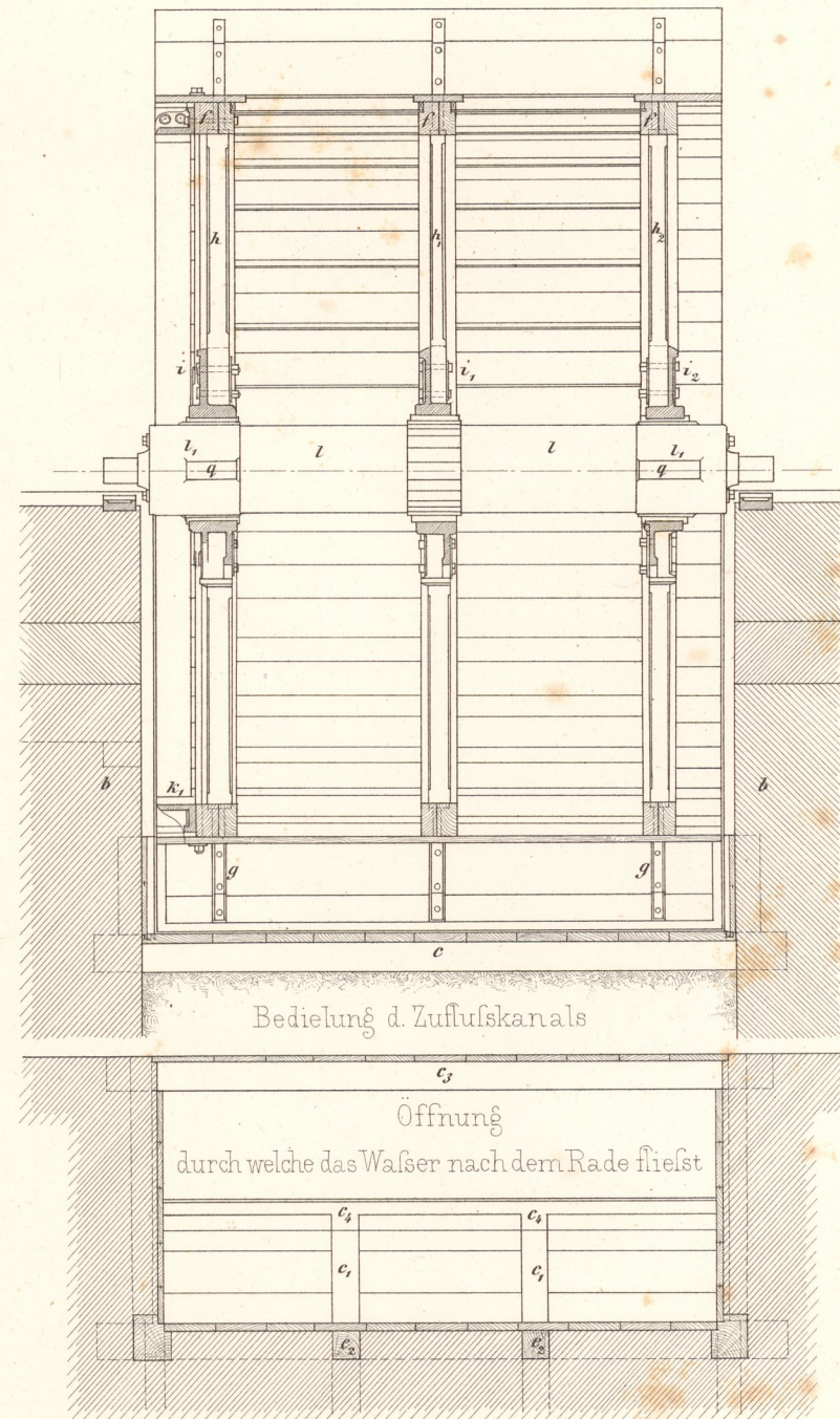
Fig. 4. Vertikalschnitt durch die Kammer vor dem Einlauf nach u.v.w.x. Fig. 1.
