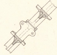
Fig. 3. Schnitt nach \alpha\beta .
