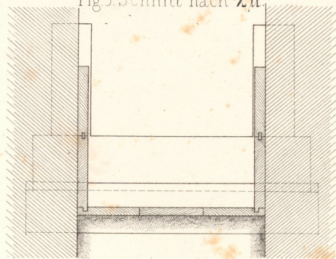
Fig. 5. Schnitt nach \lambda\mu .
