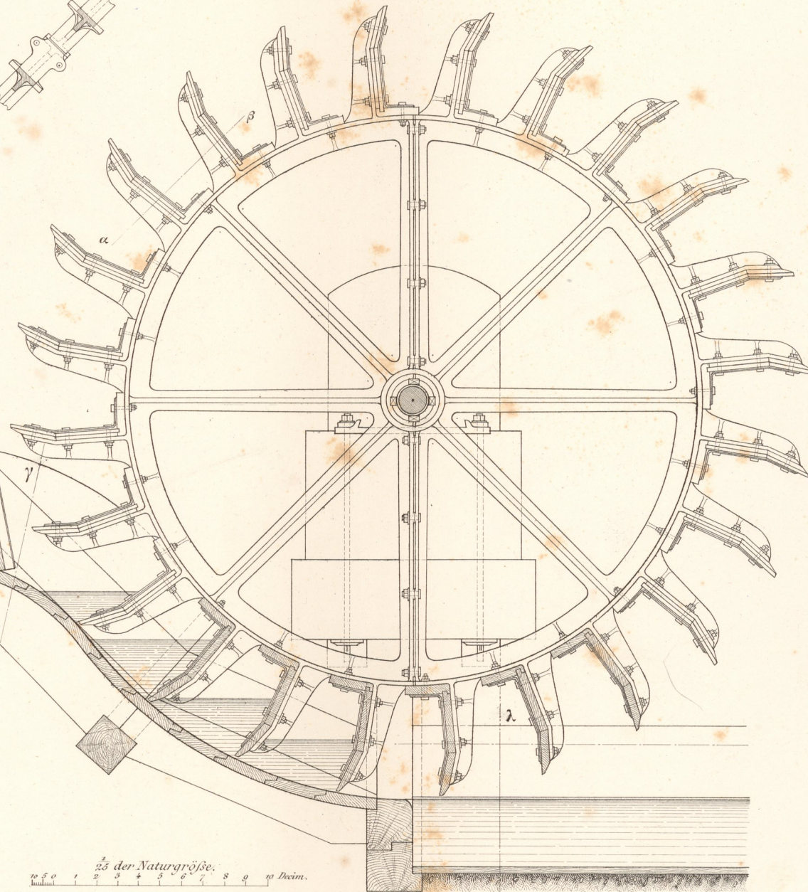
Fig. 1. Ansicht.
