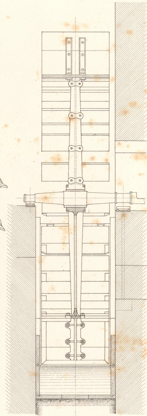
Fig. 2 Durchschnitt.
