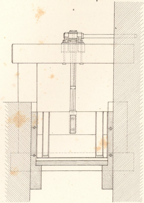
Fig. 4. Schnitt nach \gamma\delta
