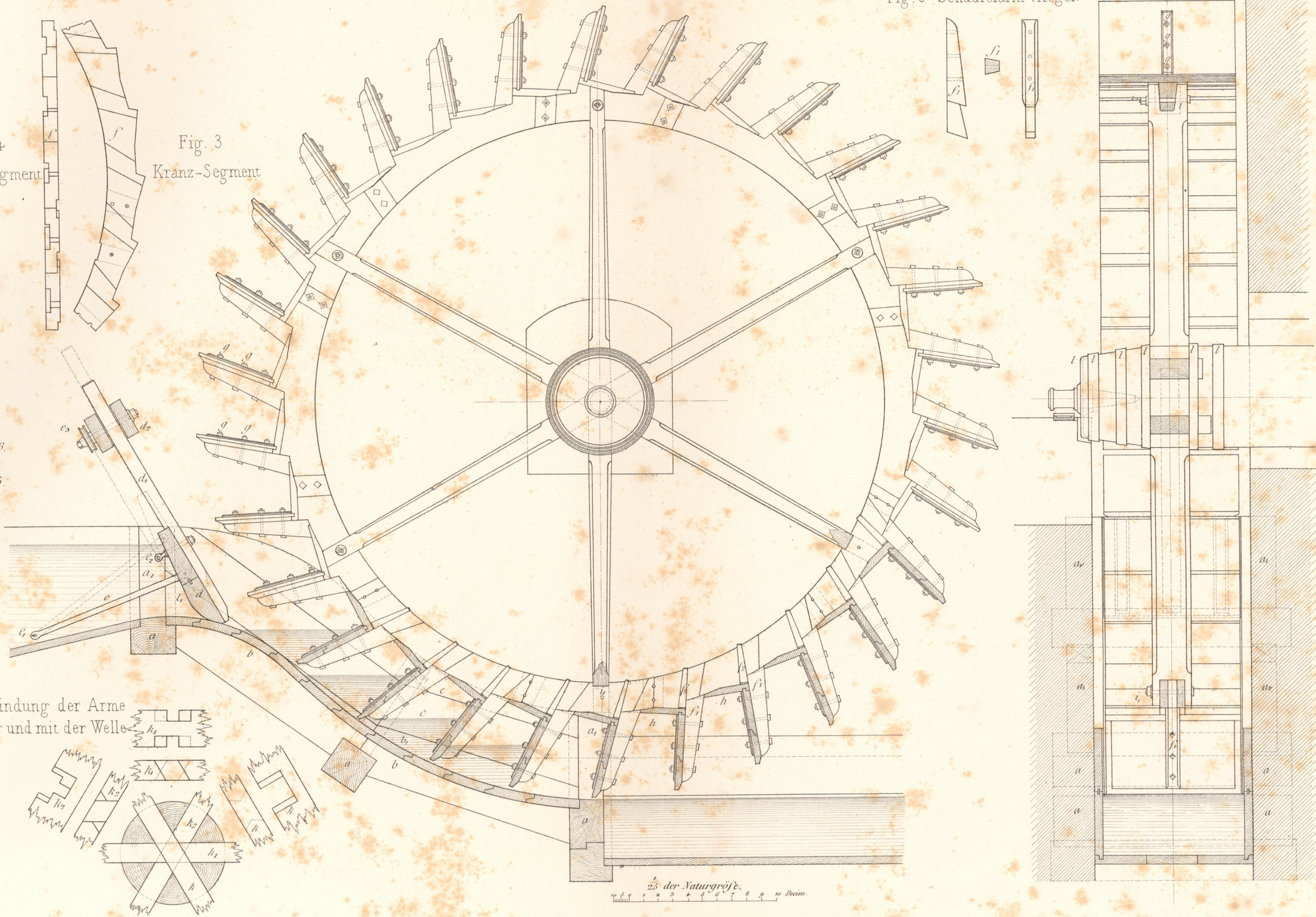
Fig. 6. Schaufelarm (Kegel)
