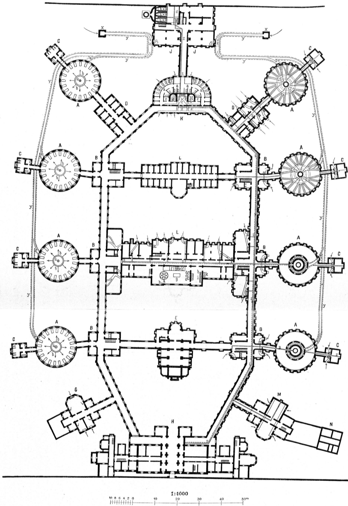
Heizungs- und Lüftungsanlage im Gasthuis Stuivenberg zu Antwerpen.
