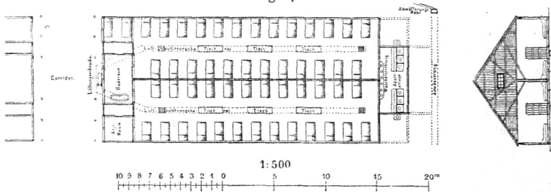
Baracke des Renkioi-Hospitals 610) .
