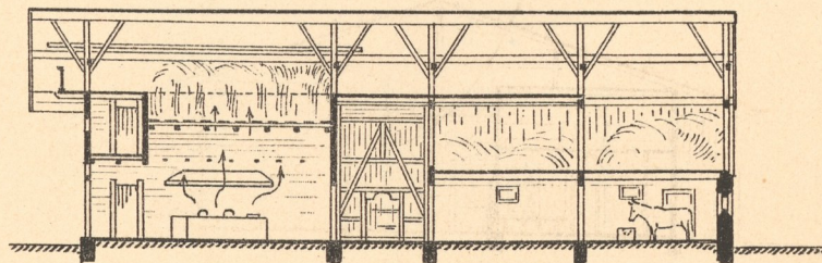
Längsschnitt nach First
