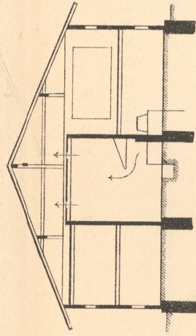
Querschnitt SS.
