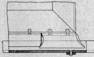
Pflugförmig gebogenes Winkelblech am unteren Rande des Schiebetores, zum Aus- räumen der Führungsebene.
