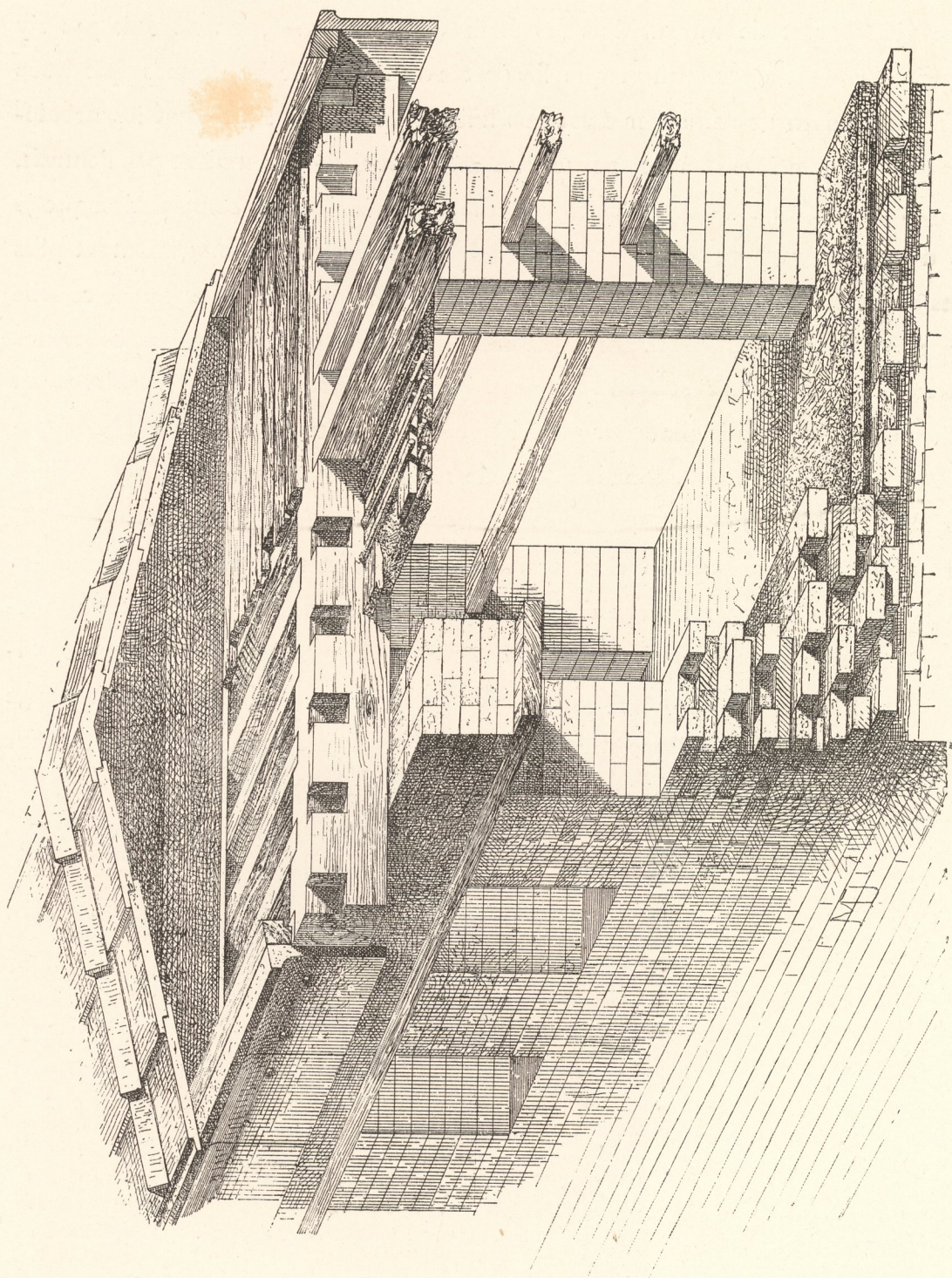
Fig. 43. — DÉTAILS DE LA COUVERTURE DES MURS DE DÉFENSE D'ATHÈNES. Restitution.
