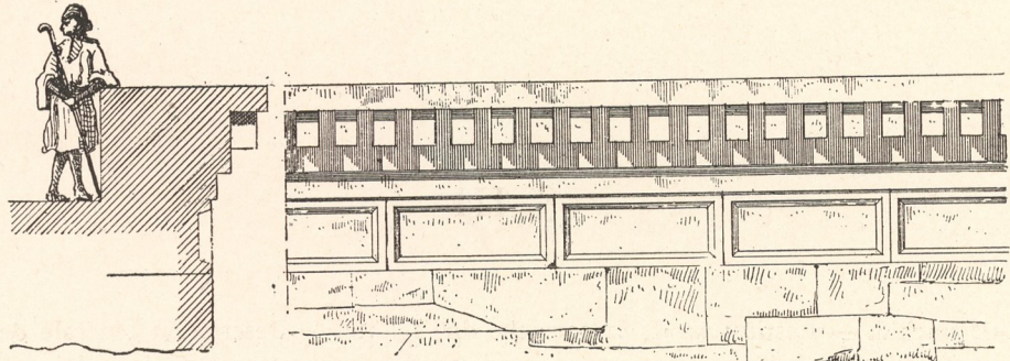
Fig. 9 et 10. — Coupe transversale et élévation du parapet restauré.
