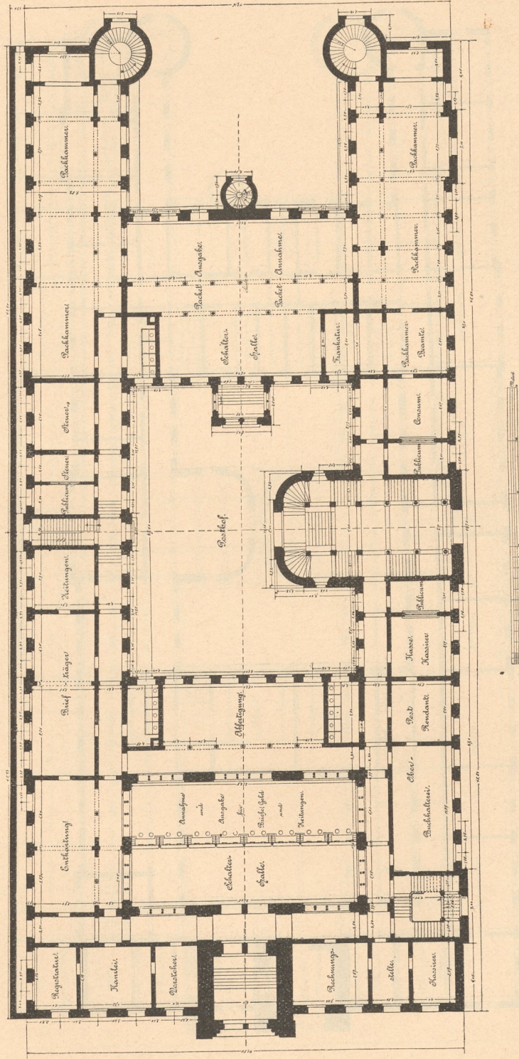
Erdegeschoss.
