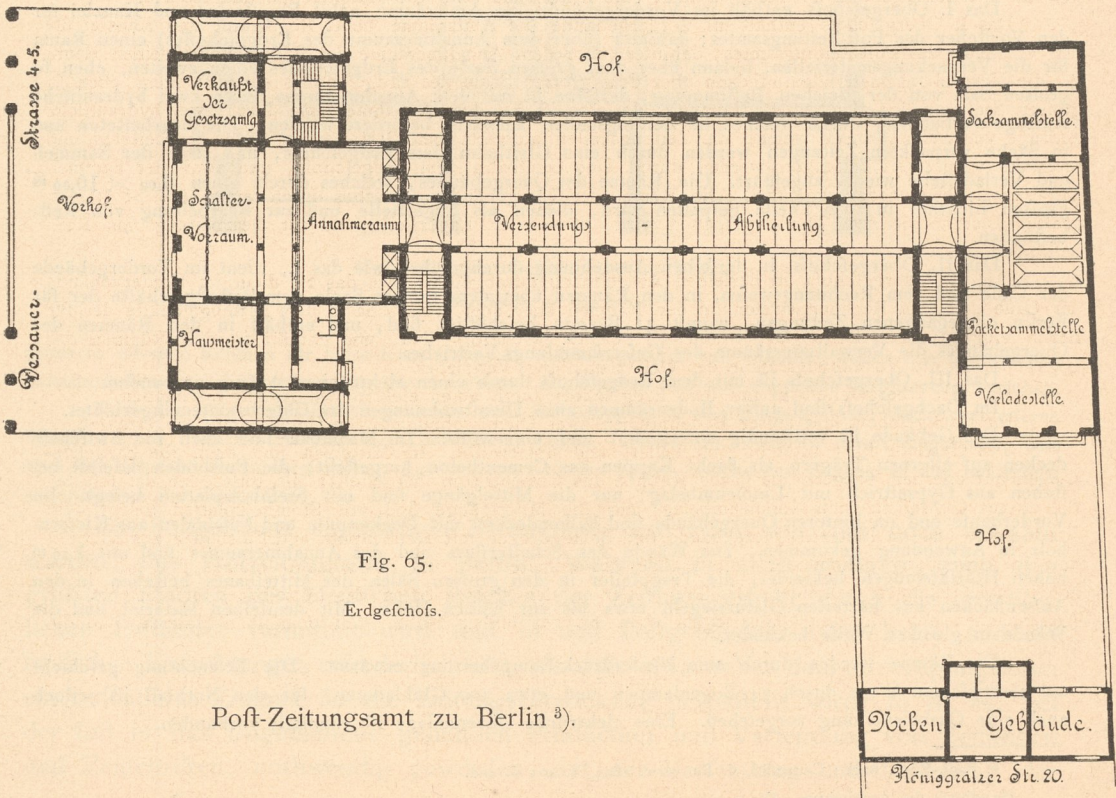
Anficht.
