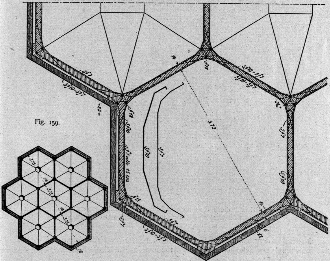
Grundriß eines Silogebäudes mit sechseckigen Zellen 63) .
