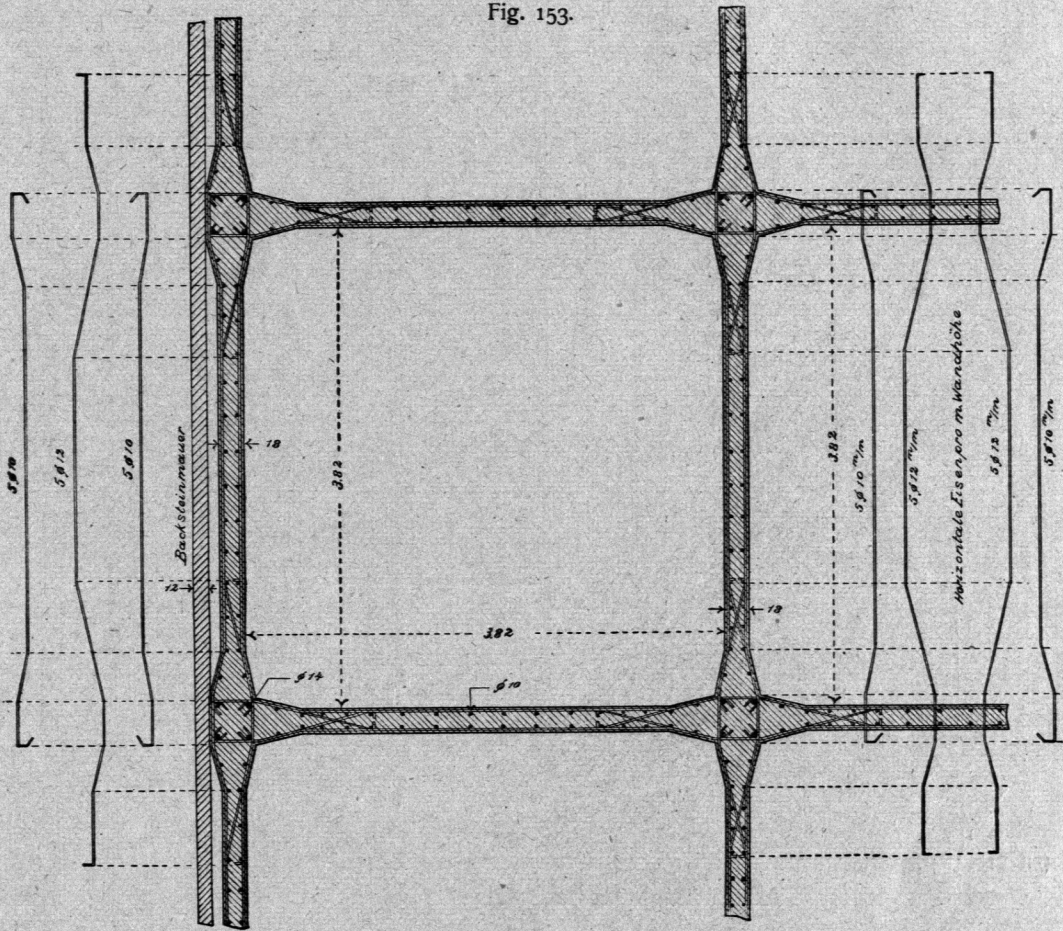
Horizontalchnitt durch rechteckige Silozellen mit Eifeneinlagen 62) .
