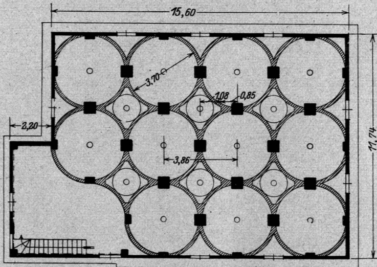
Silogebäude der Getreidemühle C. A. Meyer in Landshut. Entw. und ausgef. von der Tief- und Betonbaugesellschaft m. b. H. München.
