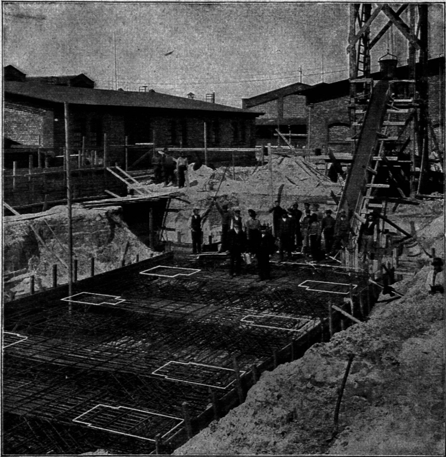
Ausführung der Eisenbetonplatte unter den Bunkerfüßen.
