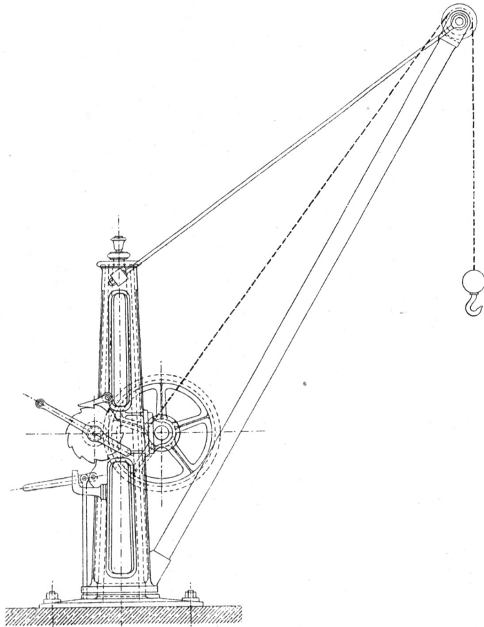
Drehkrahn in der Schweine-Schlachthalle zu Caffel.
