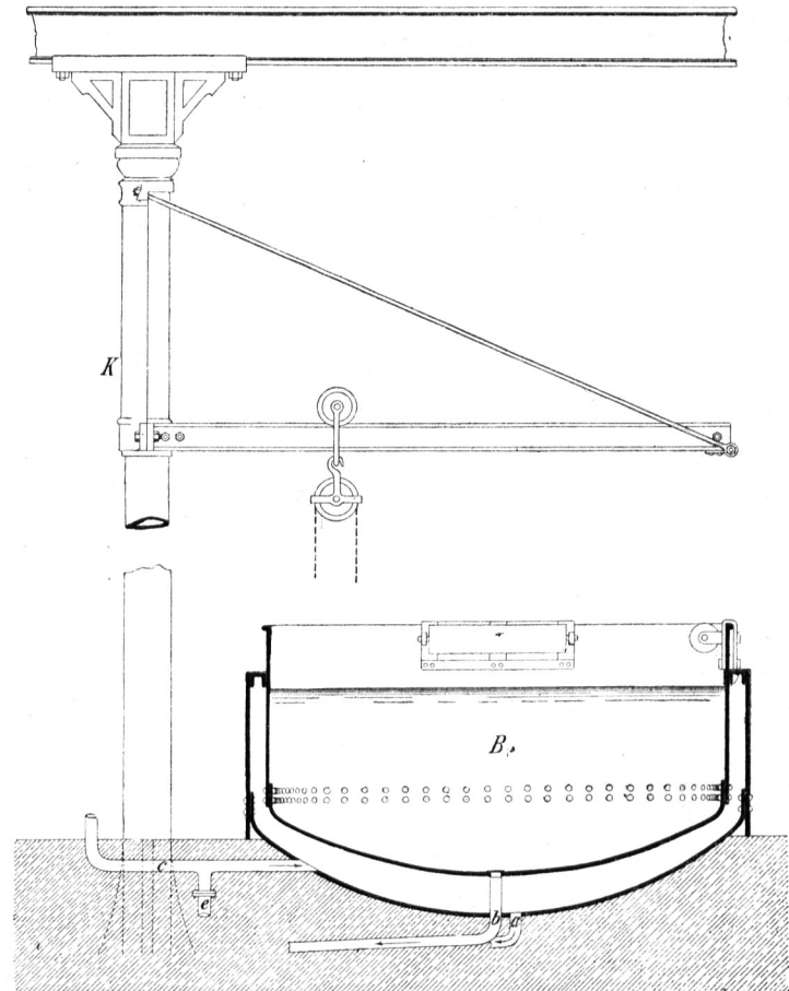
Drehkrahn mit Brühbottich in der Schweine-Schlachthalle zu Erfurt.
