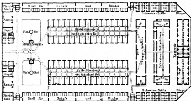
Schlachthof zu Lyon-Vaise 105) . — 1/2000 n. Gr.
