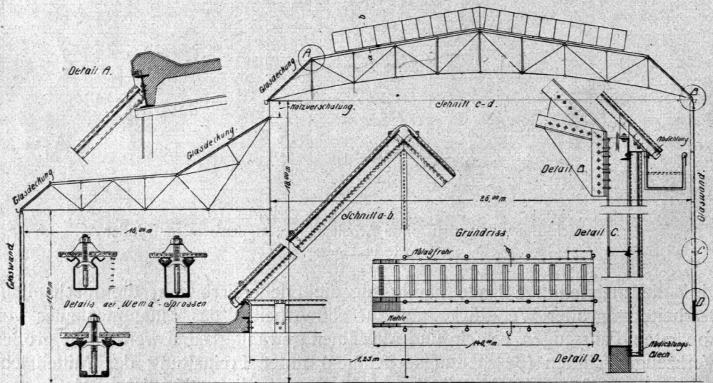
Dachbinder über einem reichbelichteten Hallenbau mit Einzelheiten der Glasdeckung.
