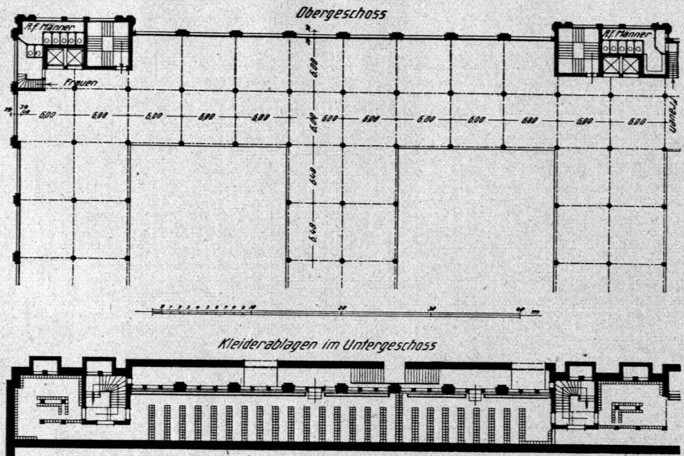
Teil des Obergeschoßgrundrisses.
