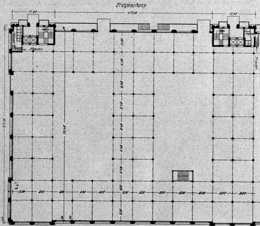
Teil des Erdgeschoßgrundrisses.
