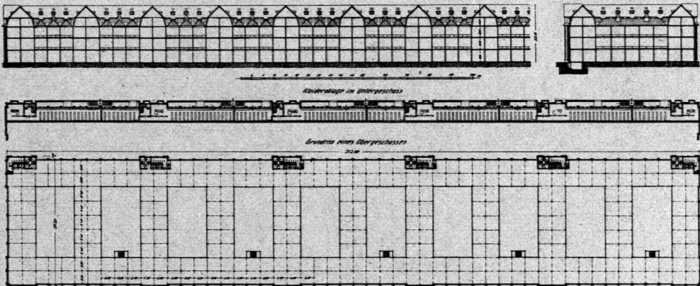
Grundrisse und Schnitte.
