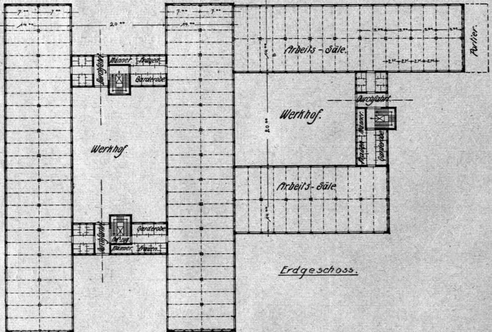
Grundriß des Erdgeschosses.
