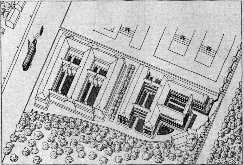
Projekt eines Werkstättenbaues für eine gemeinnützige Gesellschaft in Berlin. Schaubild.
