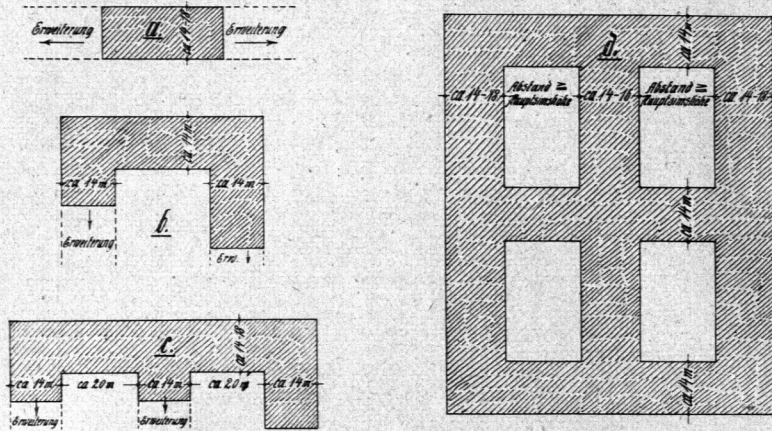
Schemafkizzen für freistehende Geschossbauten.
