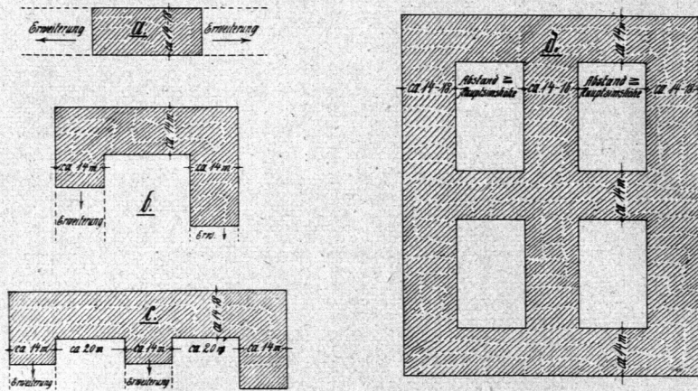
Schemakizzen für freistehende Geschossbauten.
